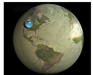
Abbildung 4 – Der maßstabsgereue kugelförmige Wassertropfen enthält das komplette Wasser der Erde (Credits: Perlman&Cook)
