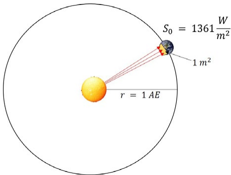
Abbildung 9 – Zur Messung der Solarkonstante bestimmt man die Leistung, die im Abstand Sonne-Erde auf 1m 2 Fläche auftrifft. (Credits: Scorza, Strähle)
